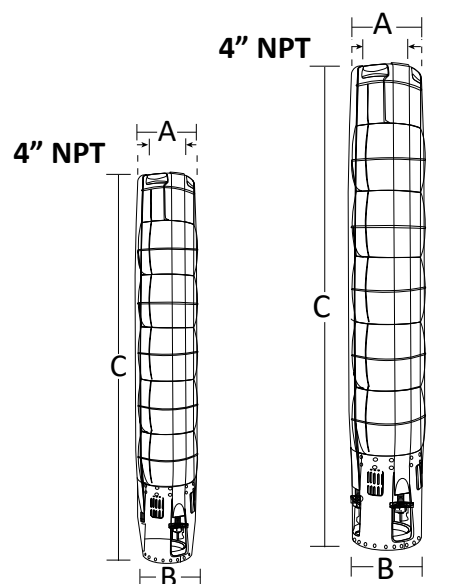
Acoplamiento NEMA 4"
